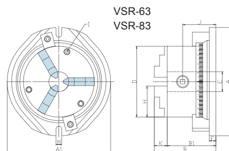
VSR-63 + VSC-6A 3JAW CHUCK VSR-83 + VSC-8A 3JAW CHUCK
